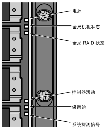
图 9.iSUM420G3 前面板指示灯
