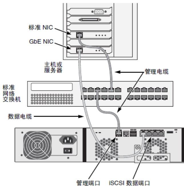
图 7.iSUM420G3 数据和管理连接
