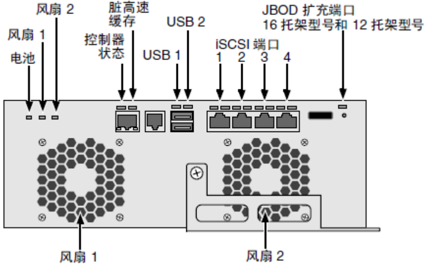
图 10 .iSUM420G3 控制器指示灯
